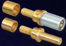
Коаксиальные
